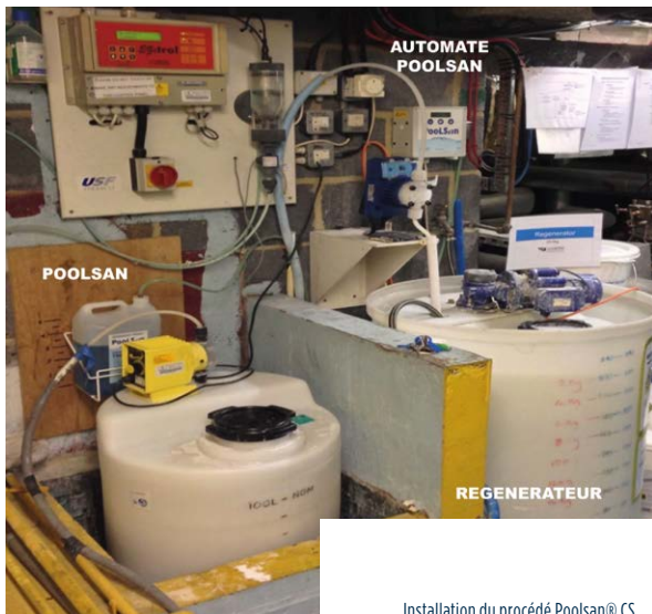
Installation du procédé Poolsan® CS
